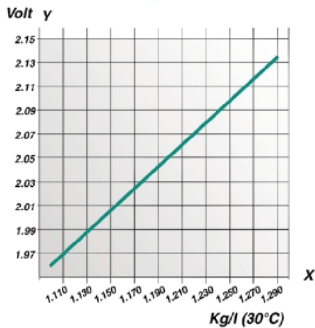
Caracteristica tensiune-densitate
