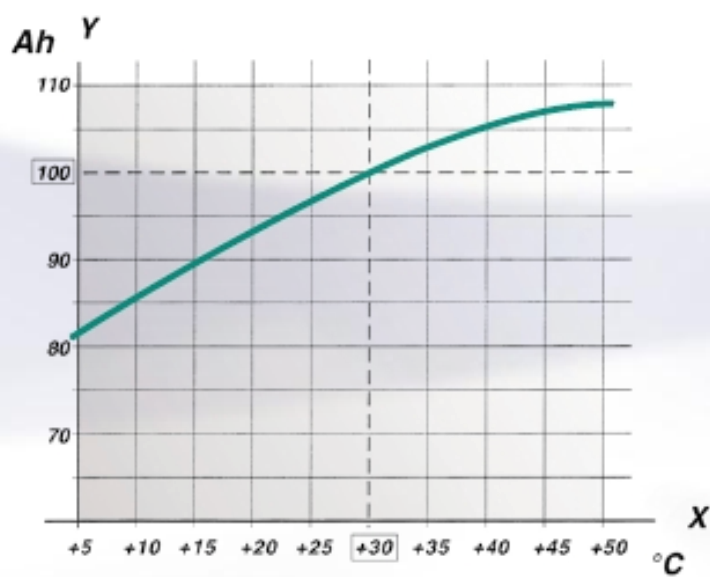
Caracteristica temperatura-capacitate
