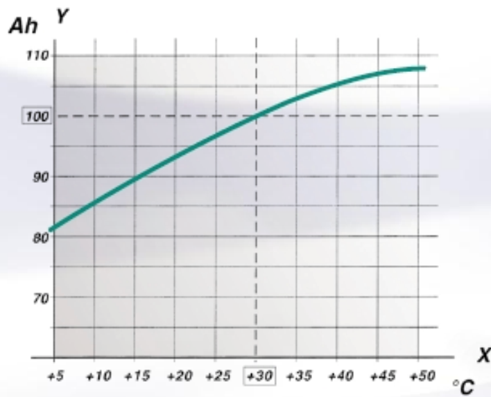
Caracteristica temperatura-capacitate
